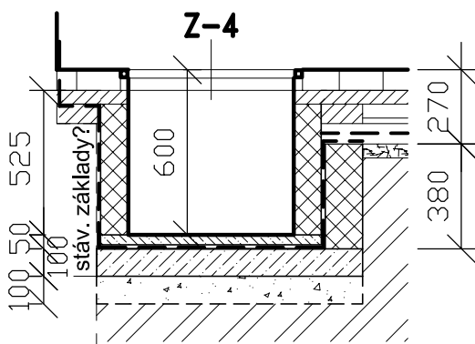
řez 1:25
