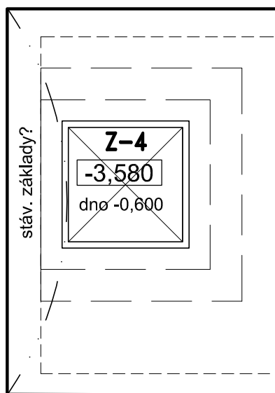
půdorys 1:25
