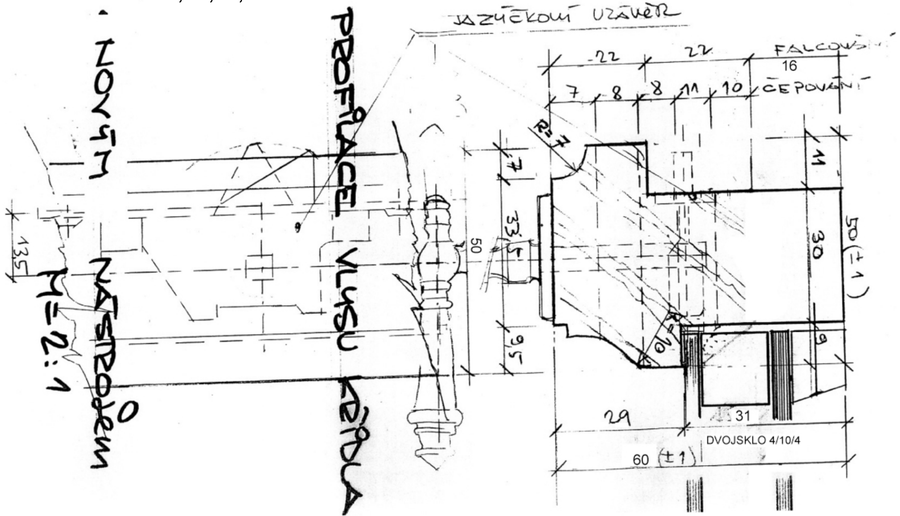
DETAIL PROFILACE VLYSU VNĚJŠÍHO KŘÍDLA U KLIČKY
