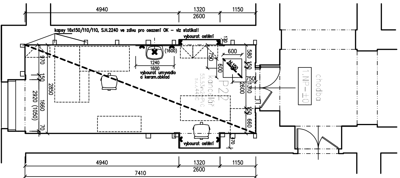
půdorys 1:50 - stávající stav
