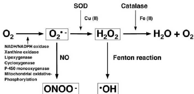
Obr. 8. Redukcí O_2 jedním elektronem vzniká reaktivní superoxid O_2^{\cdot-} . Ten je spontánně, či reakcí katalyzovanou SOD konvertován na H_2O_2 . Zejména za přítomnosti kovových iontů je pak dále Fentonovou či Haber-Weissovou reakcí oxidován na \cdot OH a reakcí katalyzovanou katalázou na vodu. O_2^{\cdot-} v malé míře reaguje s NO za vzniku ONOO^- a tím snižuje jeho dostupnost, která je pro organismus nezbytná. Peroxidázy aktivované H_2O_2 tvoří vysoce reaktivní radikál, který oxiduje NO na NO_2 a s ním reaguje na NO_2^{\cdot} , který se účastní nitrace, (převzato z Kyaw et al. 2004)
